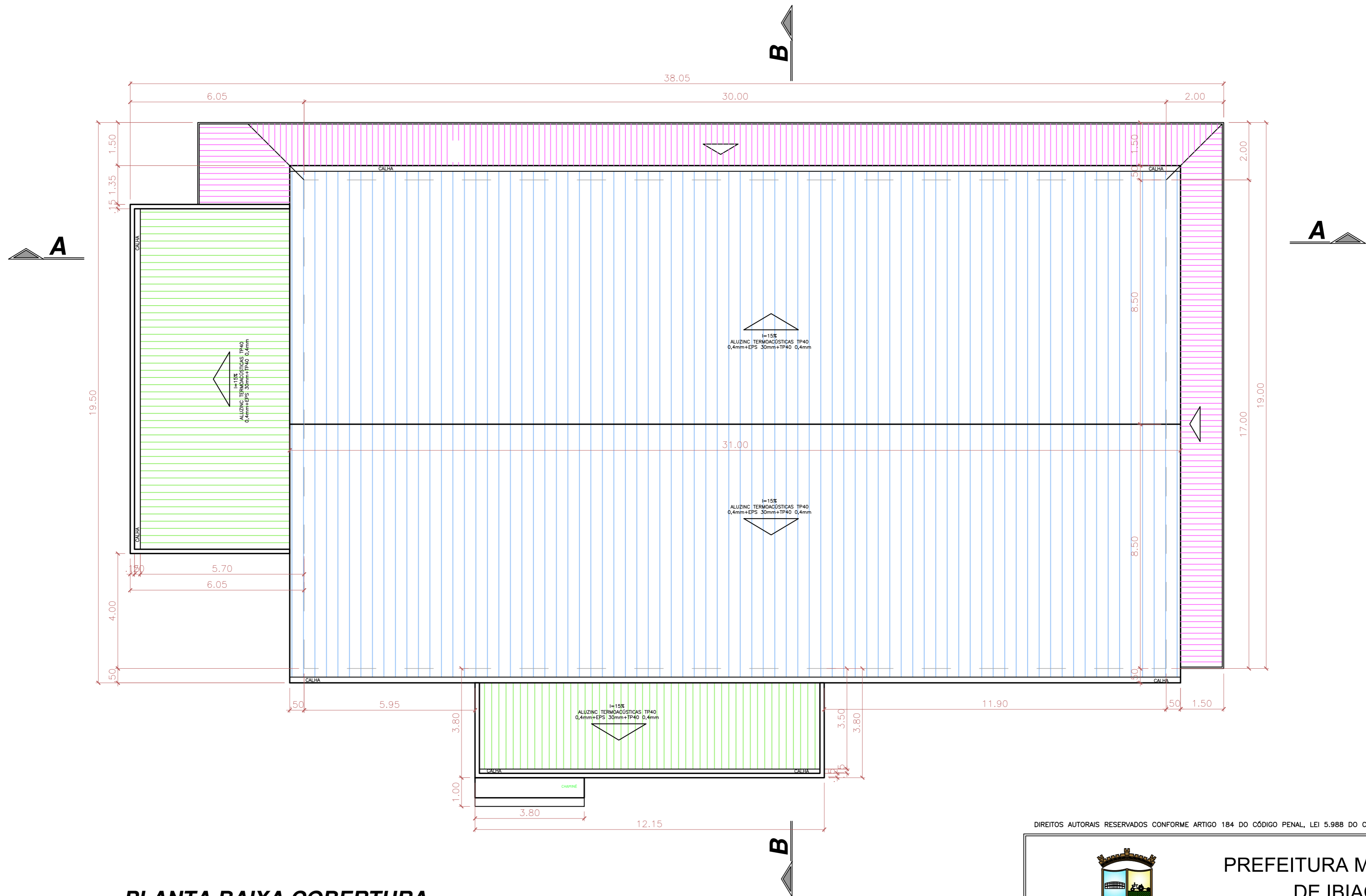
PLANTA BAIXA COBERTURA ESCALA 1:100
